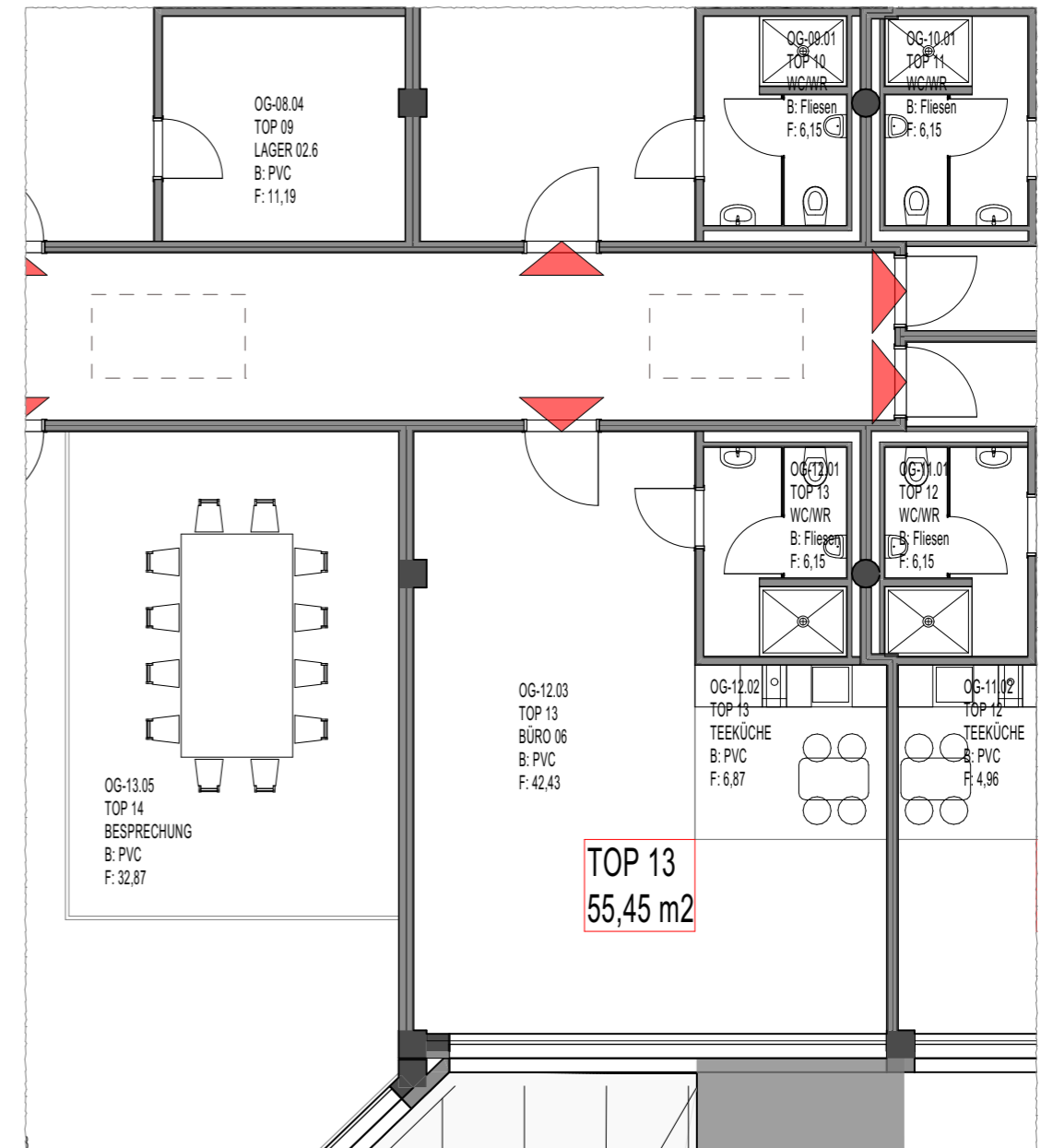
1. OG- TOP 13 Bürofläche 1:100
